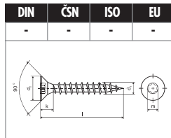
VRUT se zápusťou hlavou s hvězdicovým šestihranem TORX str. 84
