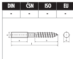
ŠROUB kombinovaný se středovým šestihranem str. 89
