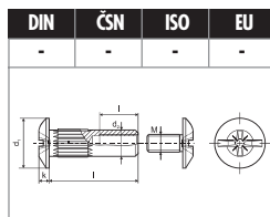
SPOJOVACÍ ČLÁNEK s hříbovou hlavou s Pozidrive + průb. drážkou str. 97
