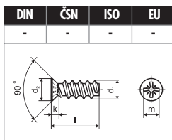
EUROVRUT se zápusťou hlavou – jemný závit str. 94
