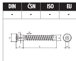
KONFIRMÁT s vnitřním šestihranem s hrubým/jemným závitem str. 95
