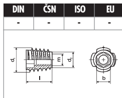
MATICE závrtná bez límce, typ E str. 99
