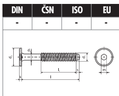
ŠROUB nábytkářský s plochou hlavou 17 mm str. 96
