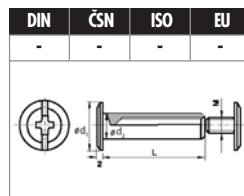
SPOJOVACÍ ČLÁNEK JCNR s Pozidrive + průběžnou drážkou str. 97
