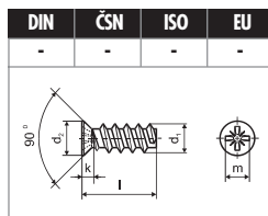
EUROVRUT se zápusťou hlavou – hrubý závit str. 94
