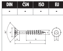
VRUT se zápusťou hlavou s hvězdicovým 6-hranem s čast. závitem str. 85
