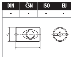
MATICE válečková vyosená str. 101
