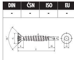
VRUT samovrtný se zápusťou hlavou s hvězdicovým šestihranem str. 86
