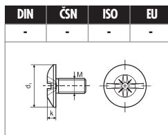
ŠROUB spojovacího článku s hříbovou hlavou s Pozidrive + průb. drážkou str. 97
