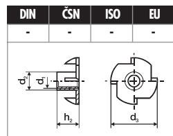
MATICE narážecí str. 98
