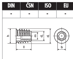
MATICE závrtná s límcem, typ D str. 99
