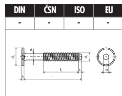
ŠROUB nábytkářský s plochou hlavou 15 mm str. 96
