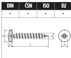
VRUT s půlkulatou hlavou s křížovou drážkou str. 88
