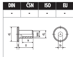
MATICE nábytkářská spojovací s plochou hlavou 17 mm str. 100
