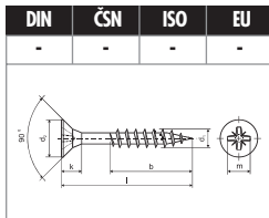
VRUT se zápusťou hlavou s křížovou drážkou s častým závitem str. 83
