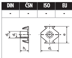
MATICE narážecí se soubky str. 98
